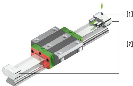
III. 5.47: Placer stålklemmer på profilsinnen
