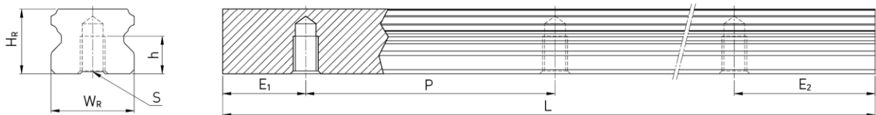
Mål på profilskinne EGR_T
