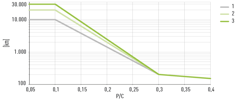
III. 8.19: Eftersmøreintervaller med smøring med fedt, en- og tosidet langtidssmøreenhed (E2/EC) for QH, QE og QW. Langtidssmøreenheden (E2/EC) er ikke tilgængelig for QW-serien.
