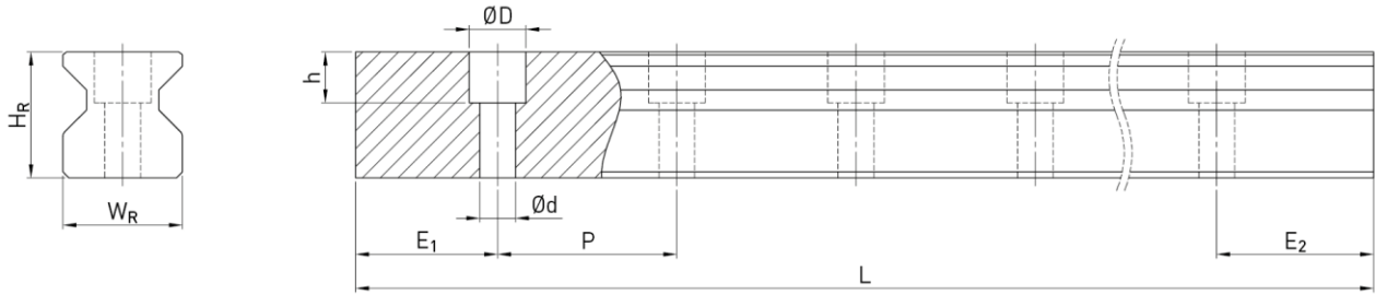
Mål på profilskinne RGR_R
