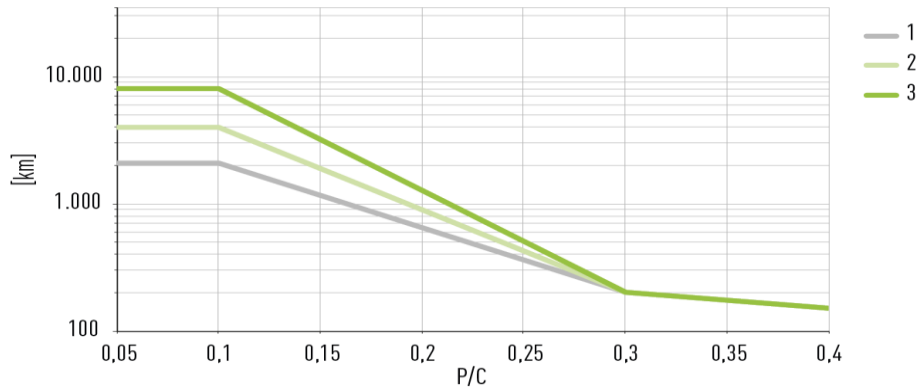
III. 8.20: Eftersmøreintervaller for smøring med fedt, ensidig og dobbeltsidet langtidssmøreenhed (E2/EF) til UR og RG.
