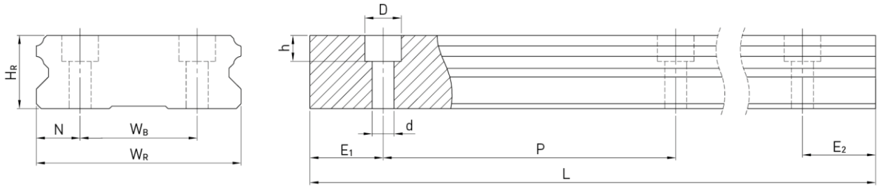
Mål på profilskinne WER_R
