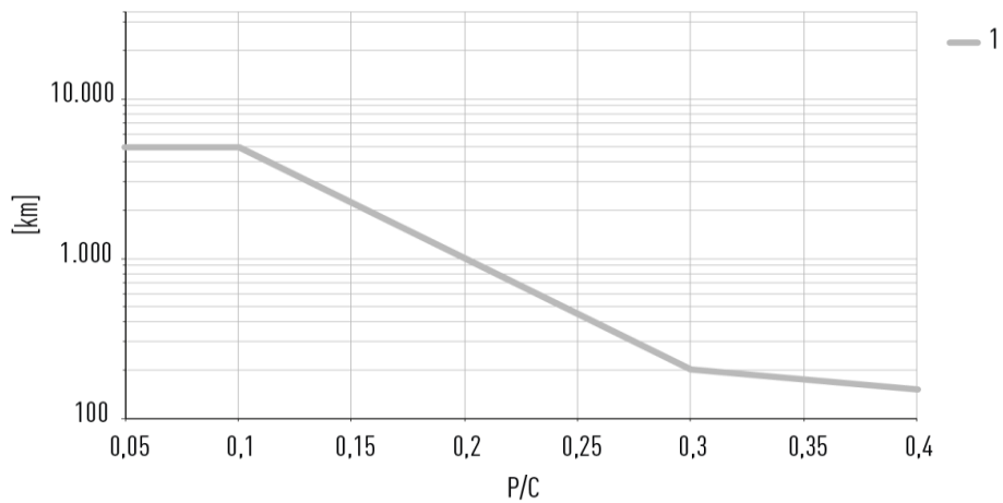
III. 8.21: Eftersmøreintervaller for smøring med fedt, ensidig og dobbeltsidet langtidssmøreenhed (E2/EC) til QR. Langtidssmøreenheden (E2/EC) er ikke tilgængelig for QR-serien.
